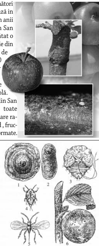
(Quadraspidiotus perniciosus Comst.): 1 - scutul femelei; 2 - scutul masculului; 3 - corpul femelei; 4 - larvă (prima vîrstă) migratoare; 5 - mascul; 6 - colonii de păduchi pe scoarță, frunză și fruct de măr (după Pospelov ș. a.)
